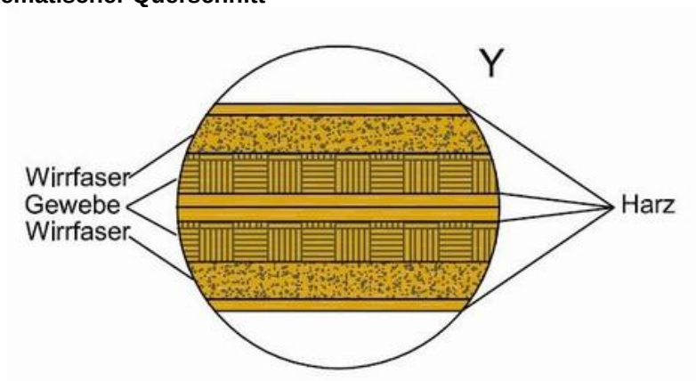
Abb. 10: Eingeharzte Glasfasergelegematte
