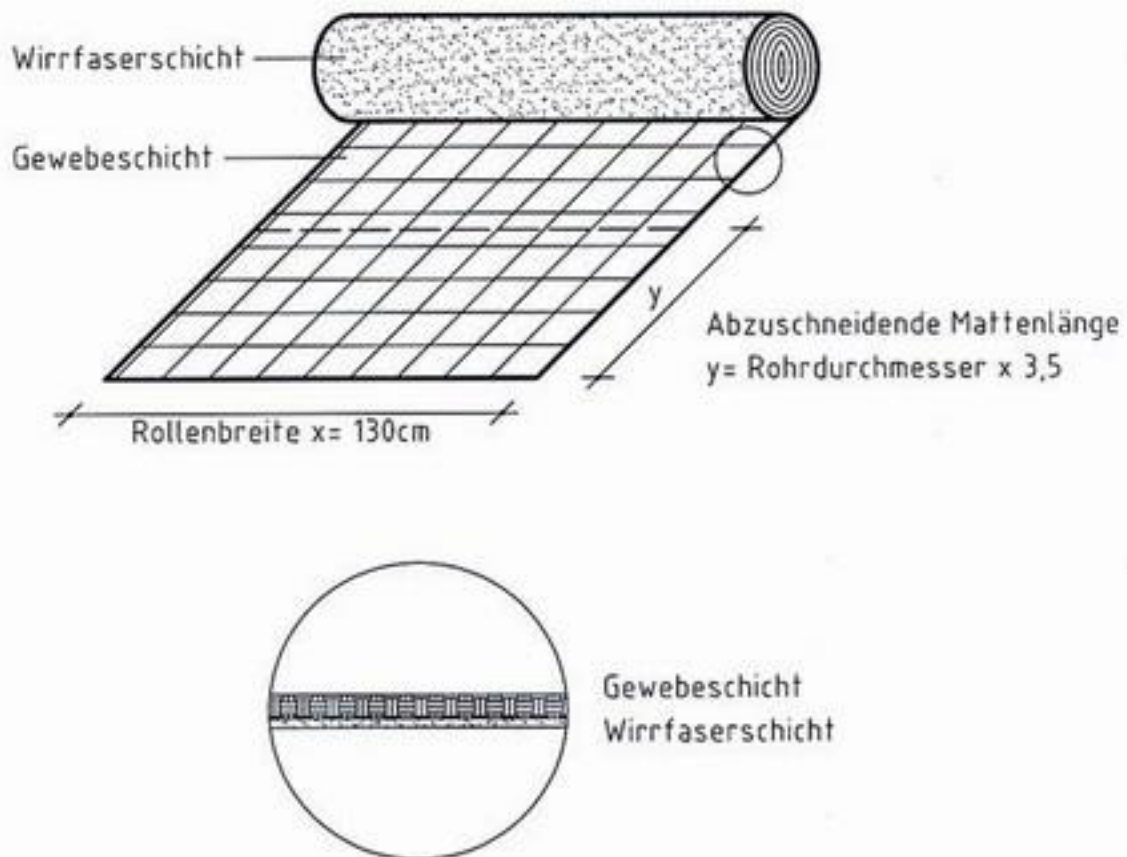
Abb. 2: 1 Wirrfaserschicht x Rollenbreite 2 Gewebeschicht y Abzuschneidende Mattenlänge
