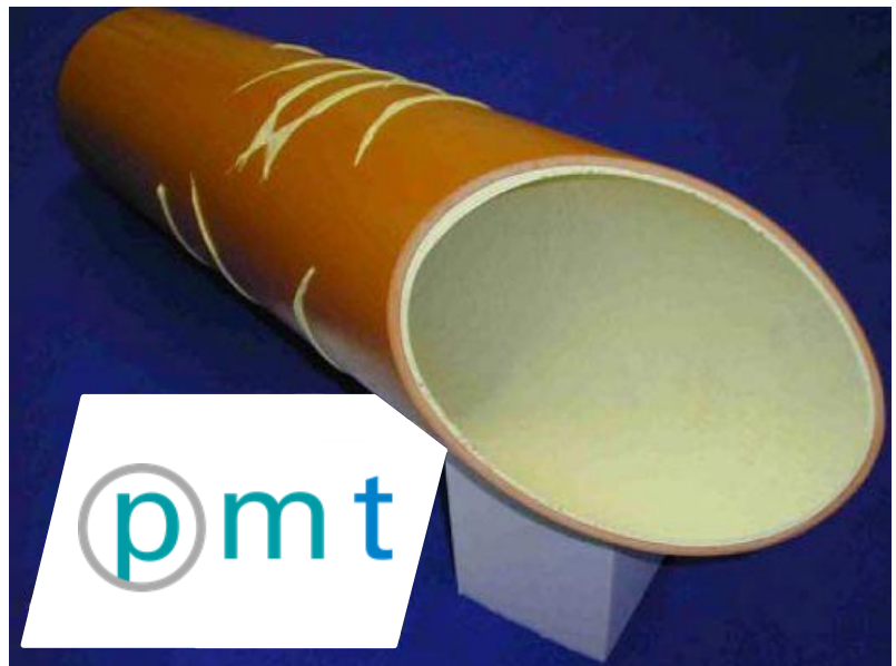
Abb. 1: Rohrleitung, saniert, SQR 2K und 3K als säure- und korrosionsbeständiger Glasfaserkomplex im Alrohr.
